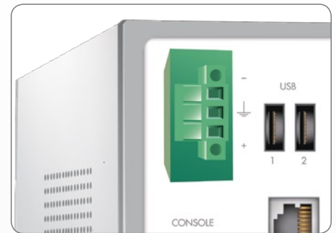
24V-Stromaufnahme Endian 4i Industrial
